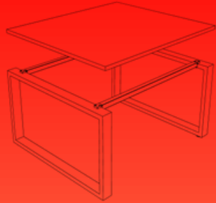
Centro de Trabajo en Espejo Arko o Kuadro
