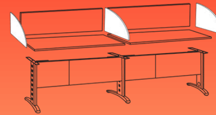
Centro de Trabajo Lineal Miami CT2.MIA | 270 → 340
